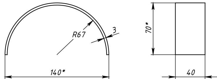
Поз.6 (Прокладка)
