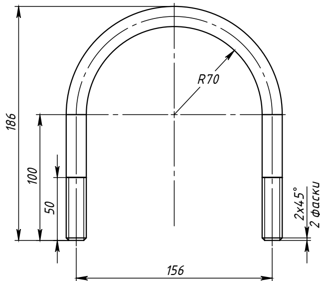
Поз.5 (Хомут)
