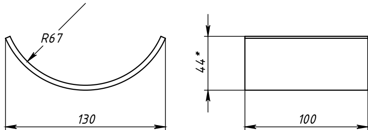
Поз.3 (Ложемент)
